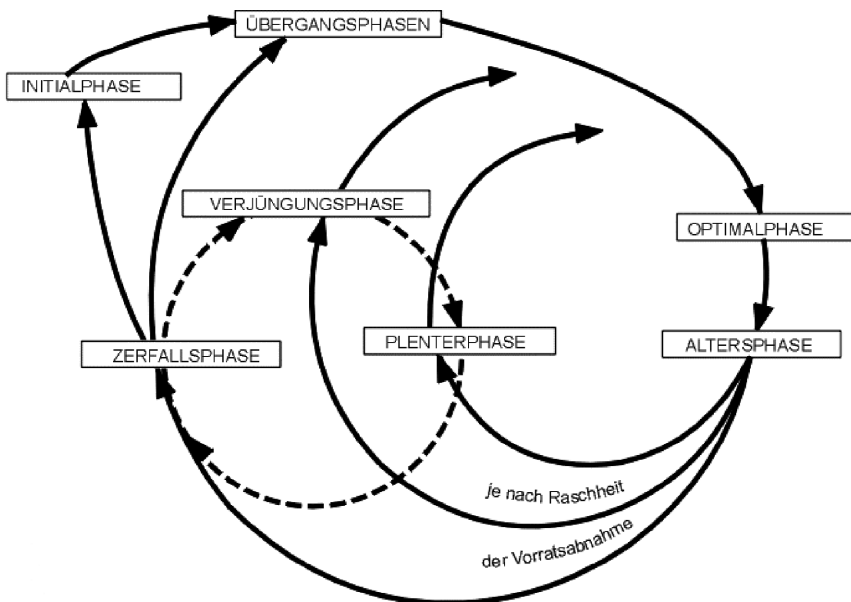
Abb. 2: Phasenfolge im urwaldartigen Bergmischwald, dargestellt am Beispiel von Urwaldresten der niederösterreichischen Kalkalpen (ZUKRIGL et al. 1963). Die Abfolge der Waldentwicklungsphasen ist weder starr noch determiniert, vielmehr kann sie an jeder Stelle durch Störungen wie Insekten-Kalamitäten, Wind- und Schneebruch unterbrochen und auf ein früheres Niveau zurückgeworfen werden.
